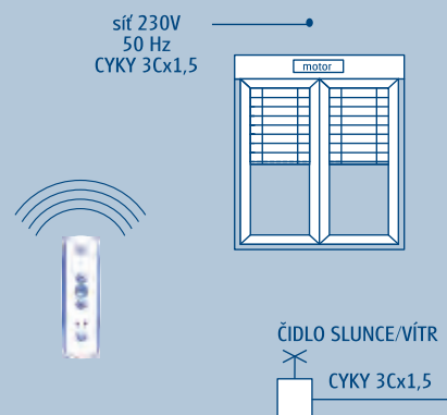
Dálkové ovládání pomocí motoru s integrovaným přijímačem Modulis Shine Receiver Plug
